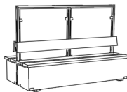
Brick Windshield Double 200 LxBxH = 1990×1060×1500 Aantal binnenbakken: 3
